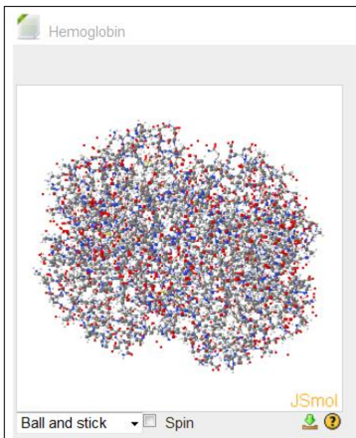
Slika 45. Prikaz molekule uporabom filtra Jmol
